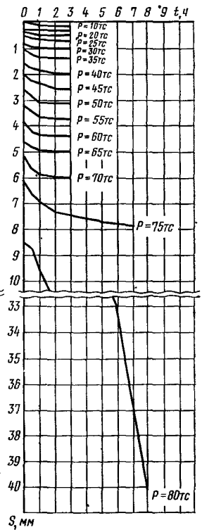
График изменения осадки сваи S во времени t (по ступеням нагрузки)
